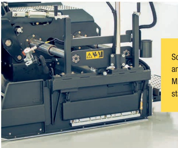
Beheizbare Seitenbleche.
