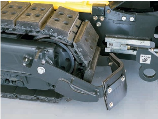
Kettenräumer garantieren einen geringen Wartungsaufwand.
