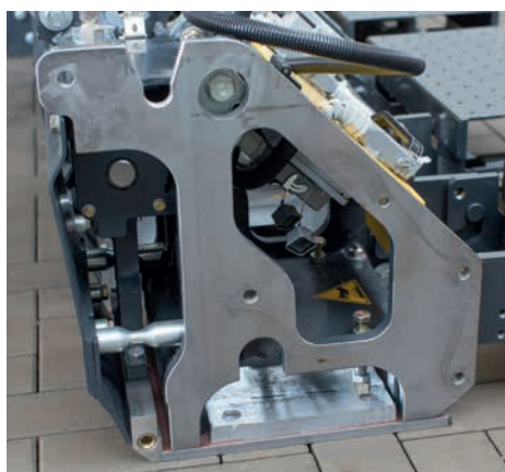
Verblüffend unkompliziert: Heizsystem mit Überwachung der Heizkreise.
